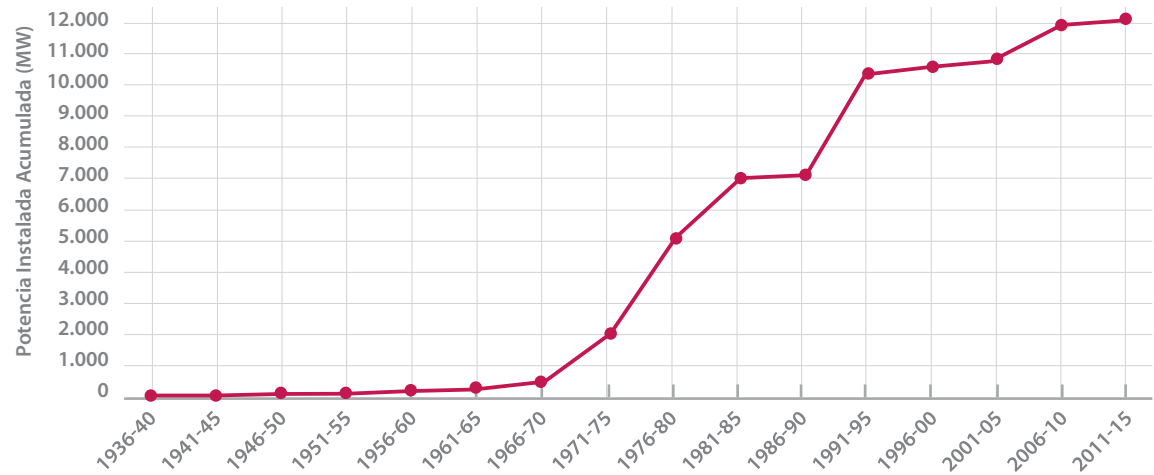
■ FIGURA 8. Evolución de la potencia hidráulica incorporada en Argentina 1936 –2013
